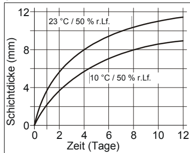
Diagramm 1: Durchhärtungsgeschwindigkeit für Sikaflex®-221
